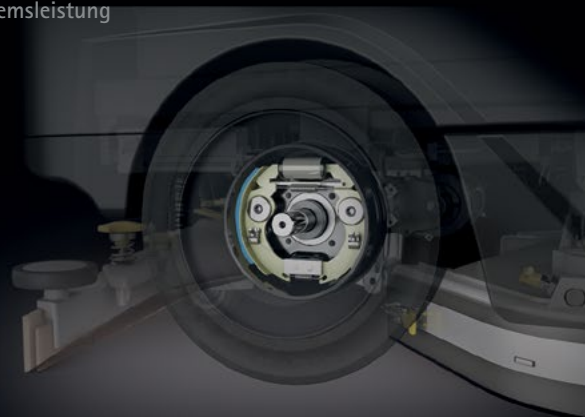
HYDRAULISCHE TROMMELBREMSEN
